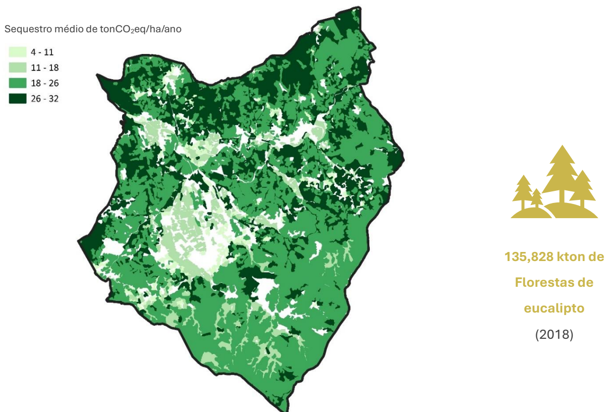
Figura 6 | Sequestro de tonCO 2 eq/ha/ano, na Lousã
