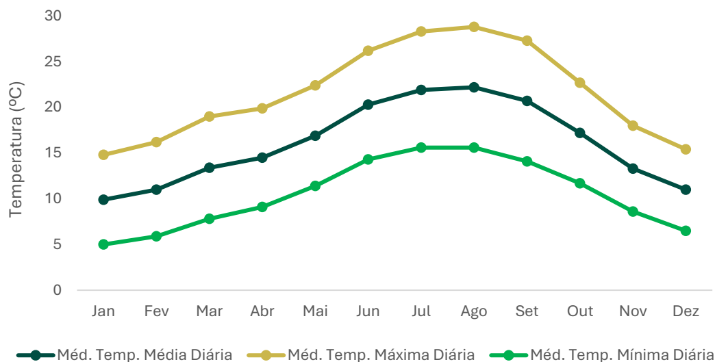
Gráfico 8 | Valores de temperatura em Coimbra, 1981-2010
